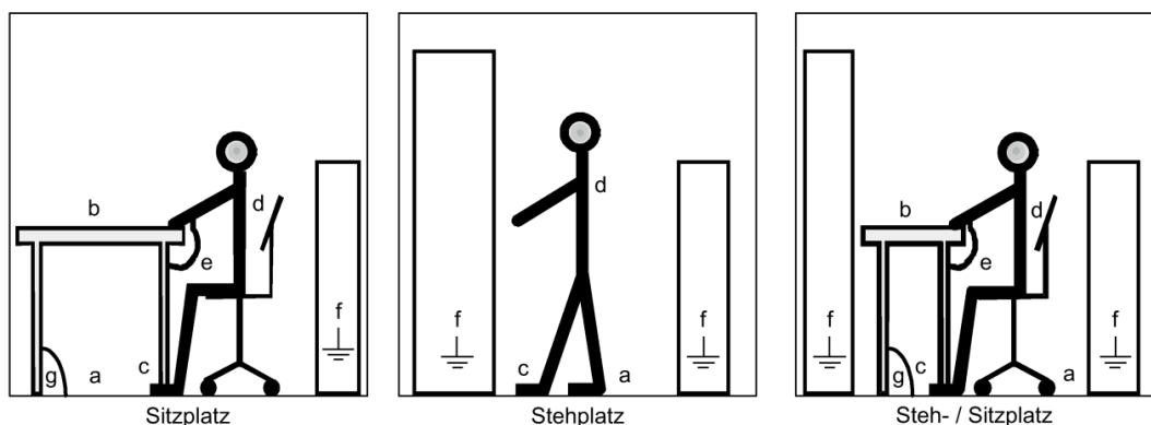
Bild 1-1 EGB-Schutzmaßnahmen
