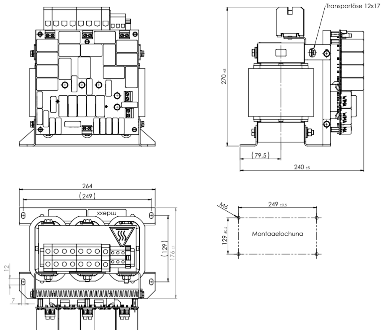
Bild 3-2 Maßblatt du/dt-Filter MTZEF051-22
